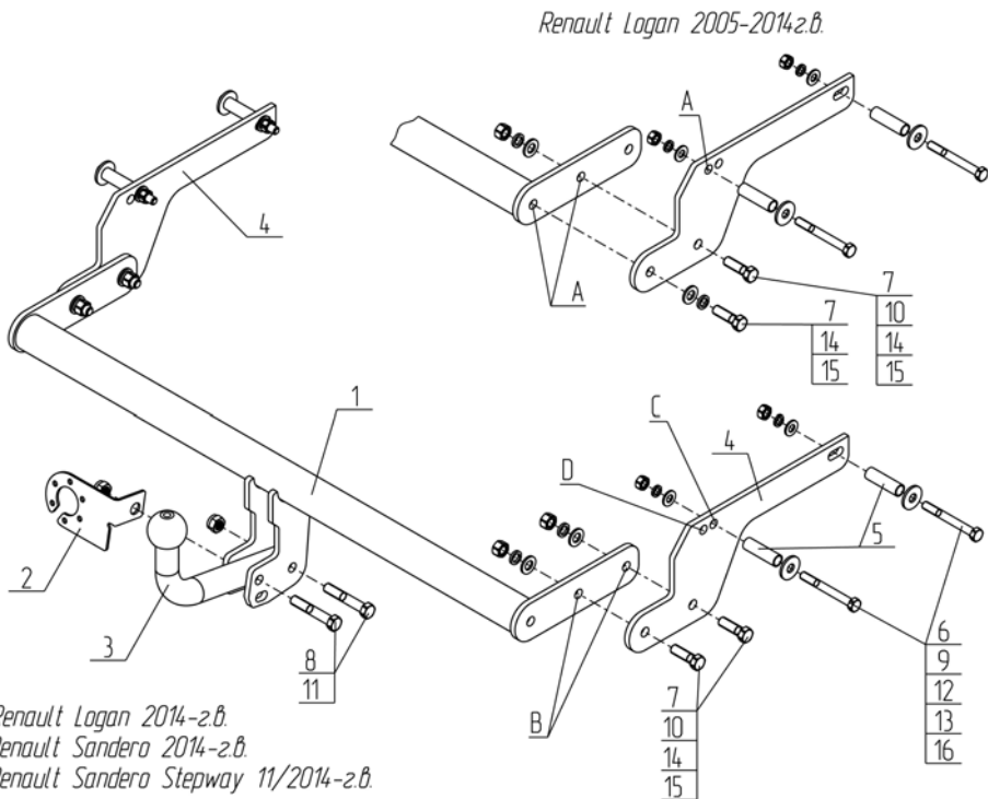
Рис.1 Установка на автомобиль
